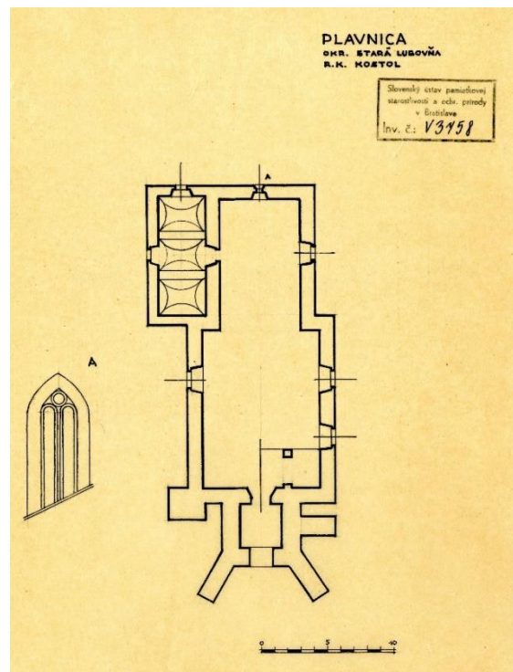
Nedatované a nesignované schematické zameranie kostola v Plavnici. Zdroj: Archív PÚ SR, nedatované (asi 50. roky 20. stor.), sign. V3758.
