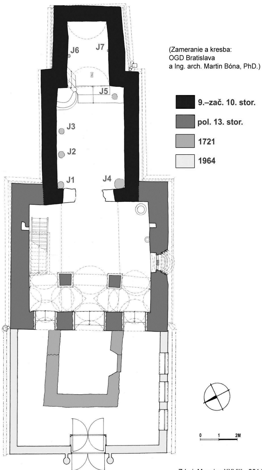
Pôdorys kostola s vývojovou analýzou
